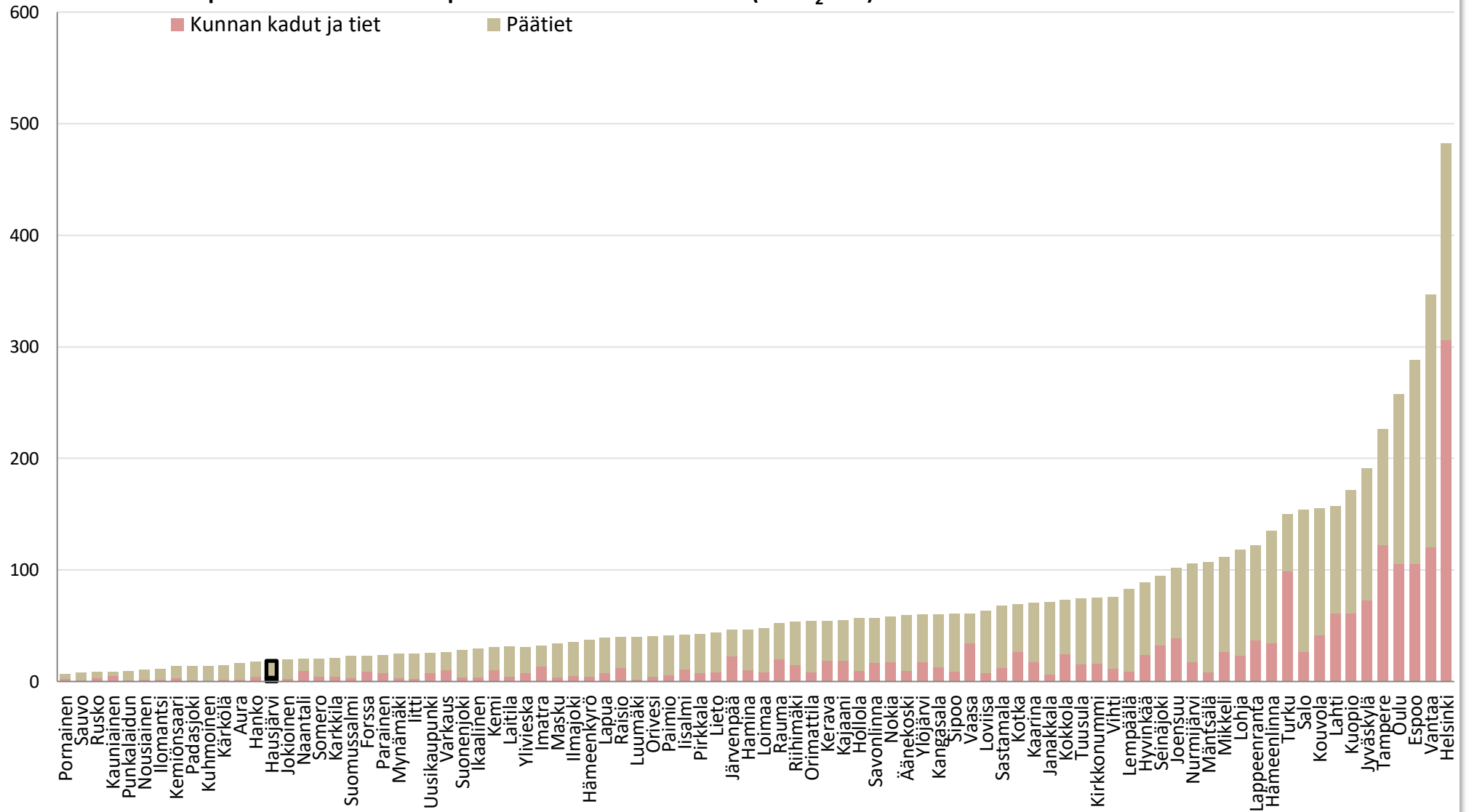
Tieliikenteen päästöt kaikissa CO2-raportin kunnissa vuonna 2020 (kt CO 2 -ekv)
