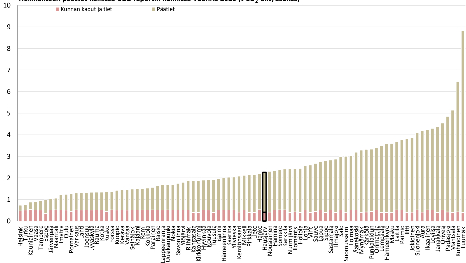
Tieliikenteen päästöt kaikissa CO2-raportin kunnissa vuonna 2020 (t CO 2 -ekv/asukas)
