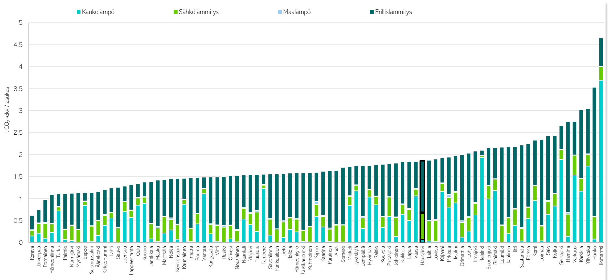
Kuva 14. Asukaskohtaiset päästöt (t CO 2 -ekv/asukas) lämmityksestä kaikissa CO 2 -raportin kunnissa vuonna 2021,
