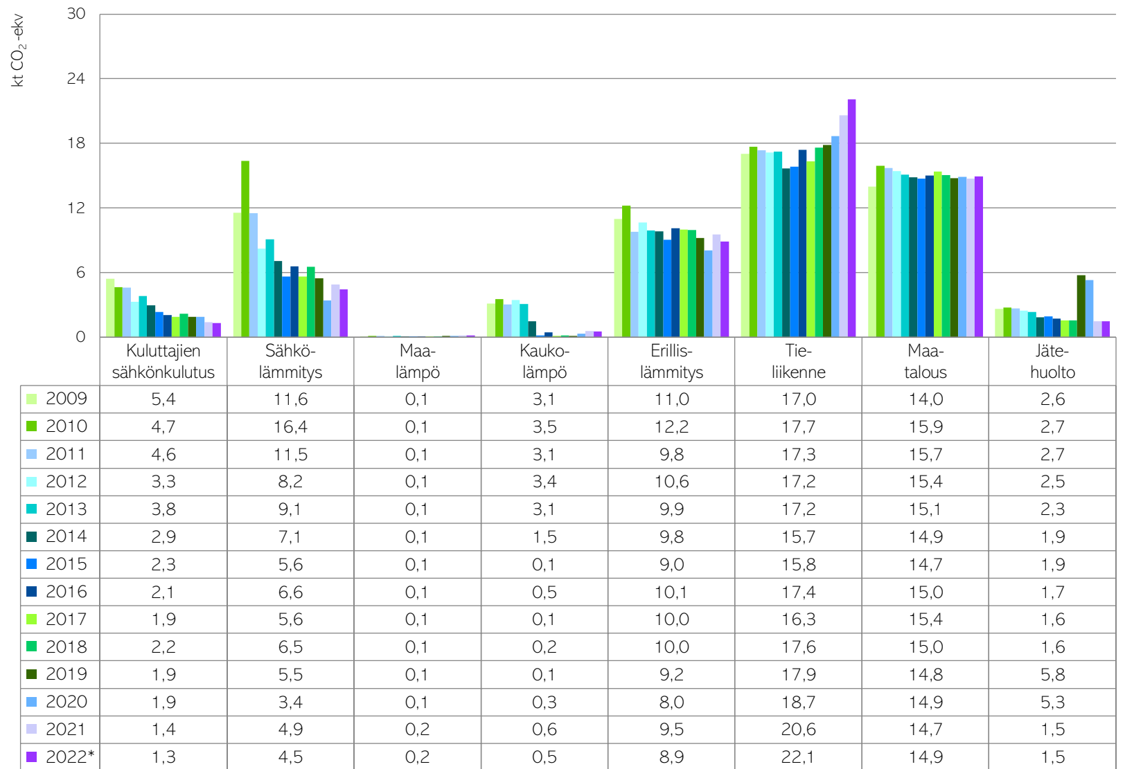
Kuva 2. Päästöt sektoreittain Hausjärvellä vuosina 2009–2022 ilman teollisuutta. Vuoden 2022 tieto on ennakkotieto.
