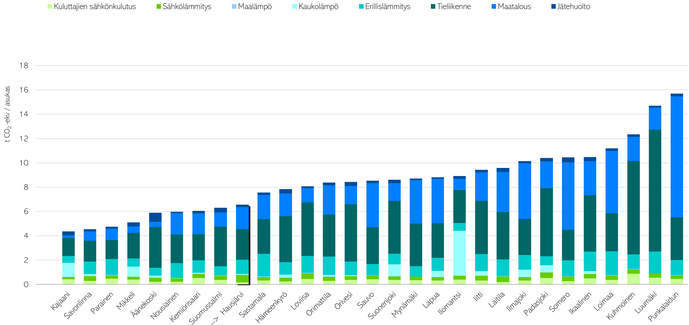
Kuva 11. Asukaskohtaisten päästöjen (t CO 2 -ekv/asukas) vertailu (ilman teollisuutta) vuonna 2021 sellaisissa CO 2 -raportin kunnissa, joissa on alle 25 asukasta maaneliökilometrillä.
