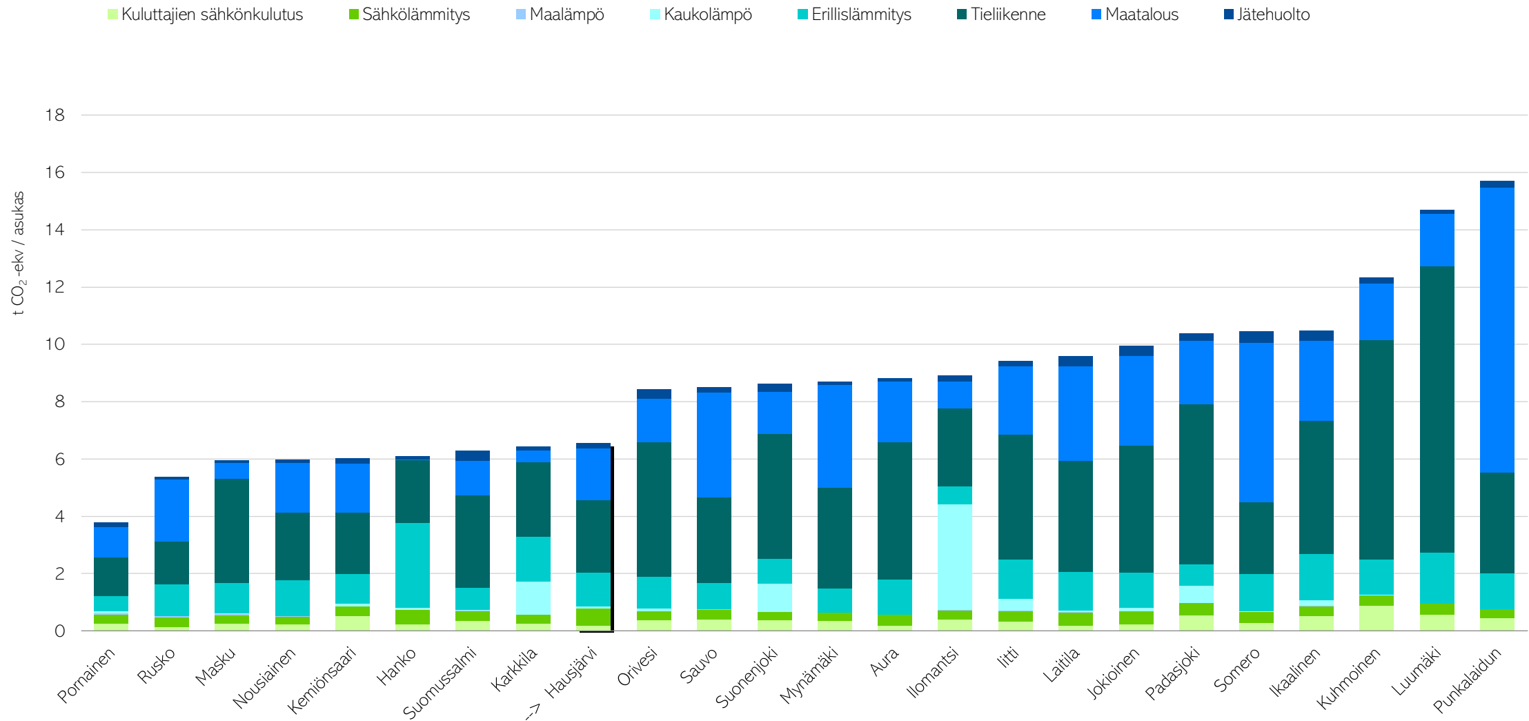
Kuva 10. CO2-raportissa mukana olevien alle 10 000 asukkaan kuntien asukaskohtaiset päästöt (t CO 2 -ekv/asukas) vuonna 2021 ilman teollisuutta.
