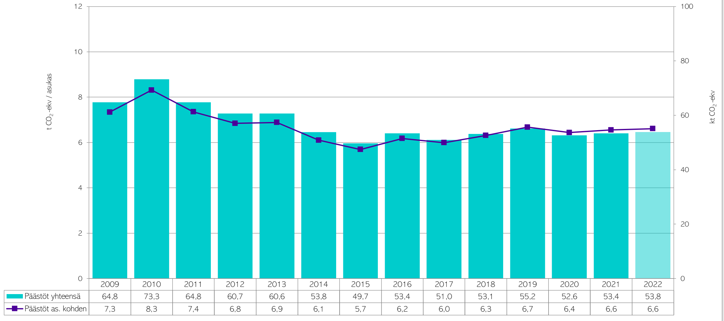
Kuva 3. Päästöt yhteensä ja asukasta kohden Hausjärvellä vuosina 2009–2022 ilman teollisuutta. Vuoden 2022 tieto on ennakkotieto.
