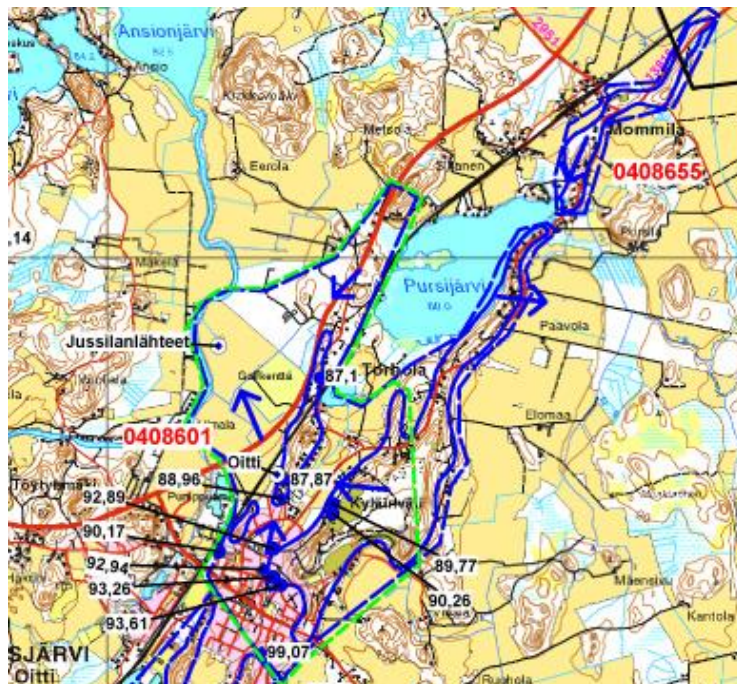
Kuva 12. Suunnittelualueella sijaitsevat Jussilanlähteet. (Ote voimassa olevan kaavan kaavaselistuksesta 2010 - Riihimäen seudun pohjavesialueiden suojelusuunnitelma, Ins.tsto Paavo Ristola)
